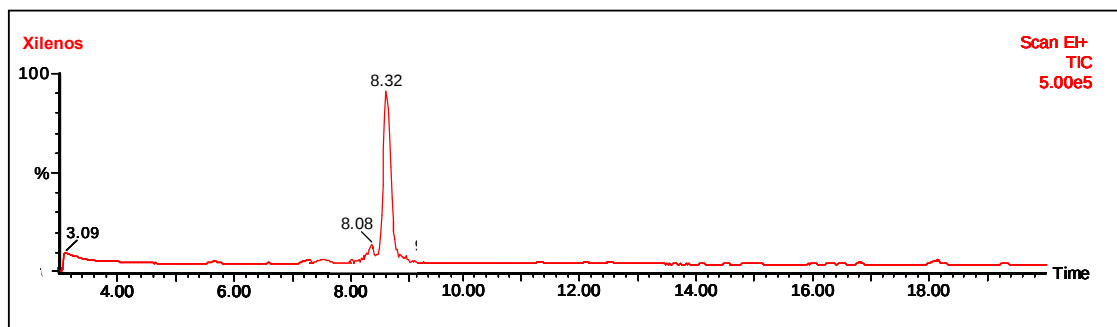
GRÁFICO 12 - Cromatograma típico dos Xilenos obtido através da cromatografia gasosa, demonstrando os sinais gerados por cada constituinte presente no sistema de olfatométrico.
