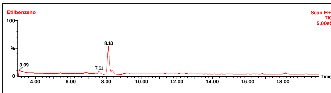
GRÁFICO 11 - Cromatograma típico do Etilbenzeno obtido através da cromatografia gasosa, demonstrando os sinais gerados por cada constituinte presente no sistema de olfatométrico.
