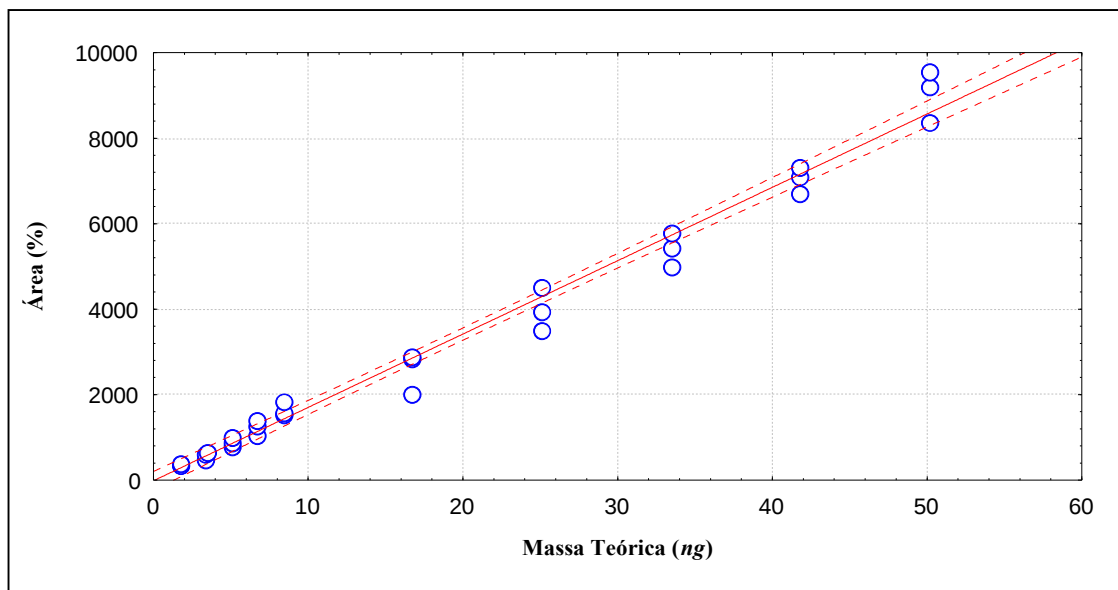
GRÁFICO 4 - Diagrama de dispersão e a reta de regressão da massa ( ng ) versus a área (%) para o Tolueno.
