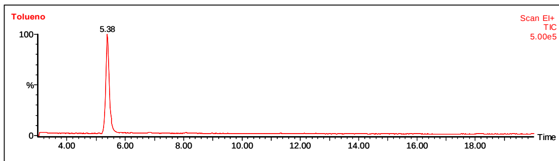
GRÁFICO 10 - Cromatograma típico do Tolueno obtido através da cromatografia gasosa, demonstrando os sinais gerados por cada constituinte presente no sistema de olfatométrico.
