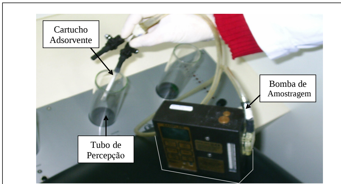
FIGURA 9 - Amostragem ativa dos compostos TEX no olfatômetro ODILE MC 2000.
