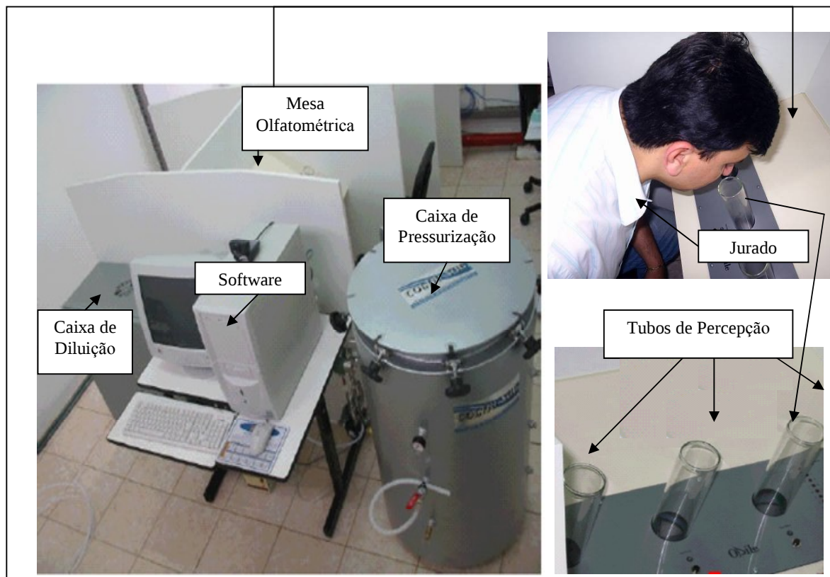
FIGURA 8 - Vista Superior do Olfatômetro de diluição dinâmica ODILE MC .
