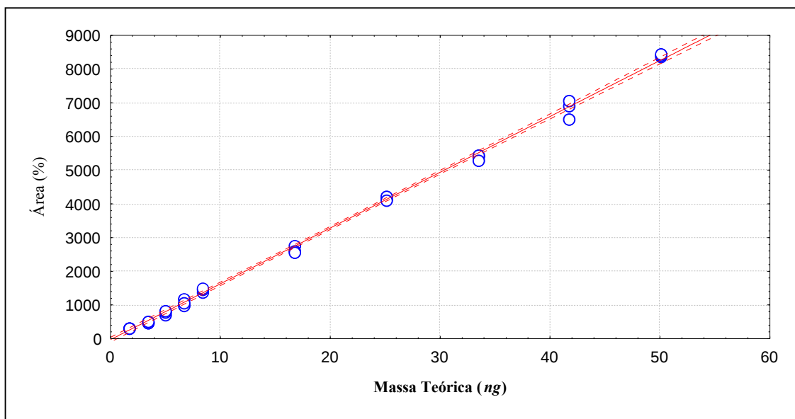
GRÁFICO 5 - Diagrama de dispersão e a reta de regressão da massa (ng) versus a área (%) para o Etilbenzeno.
