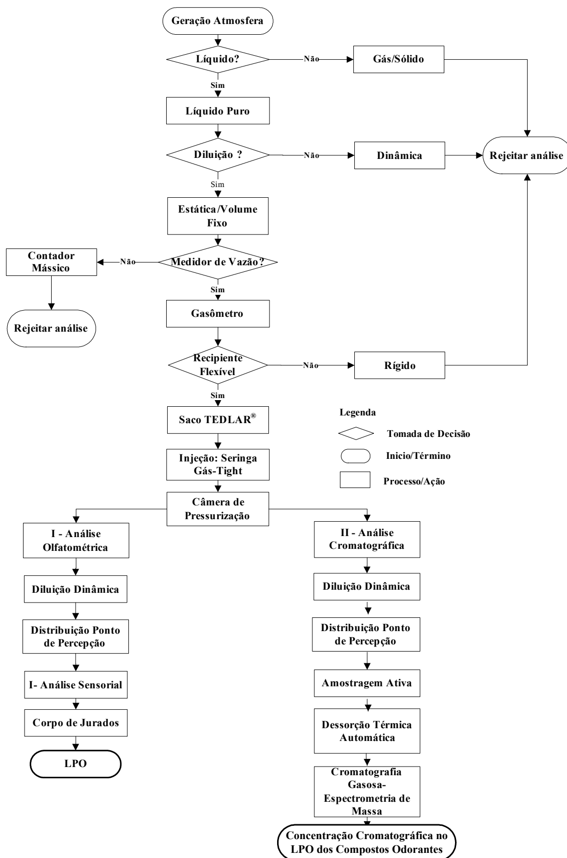
FIGURA 11 - Modelo de fluxograma para investigação do LPO de compostos odorantes a partir de um sistema de geração de atmosferas.
