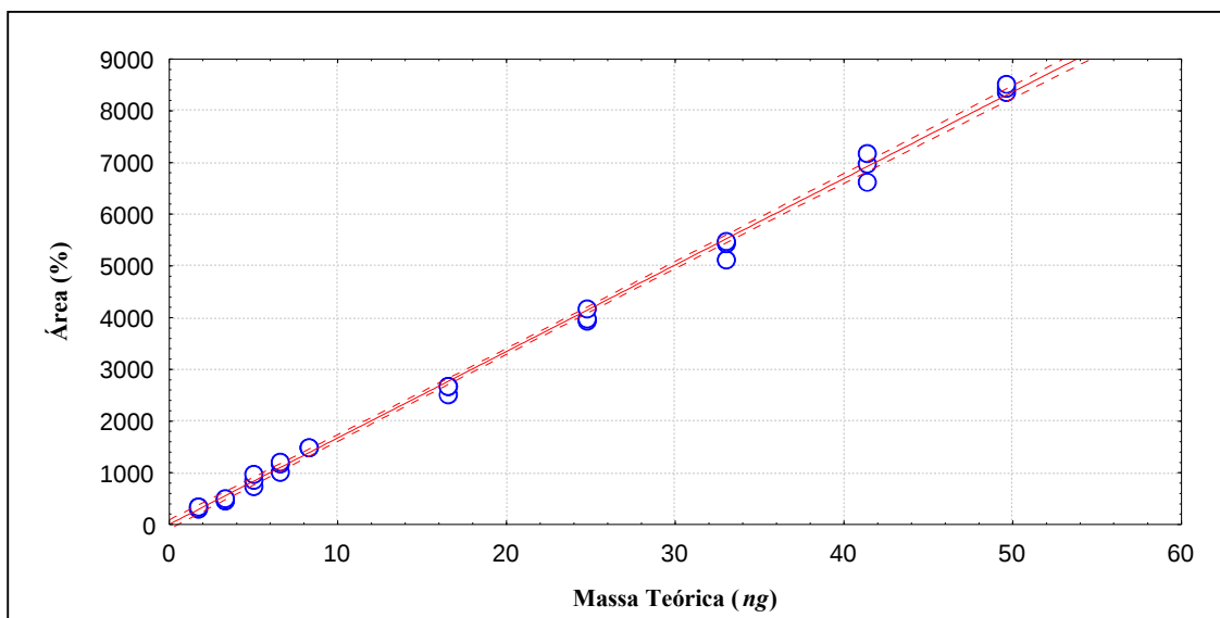
GRÁFICO 6 - Diagrama de dispersão e a reta de regressão da massa (ng) versus a área (%) para os Xilenos.
