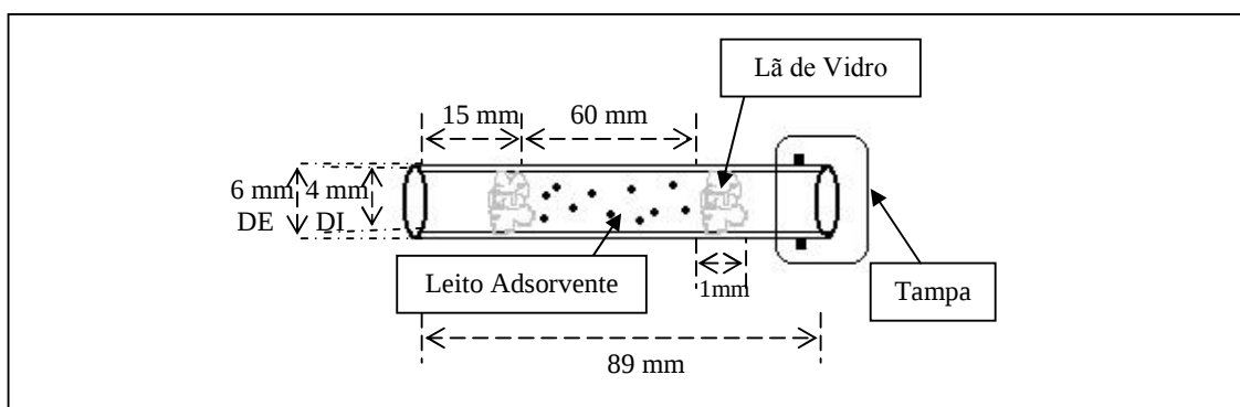
FIGURA 4 - Desenho esquemático de um cartucho adsorvente.
