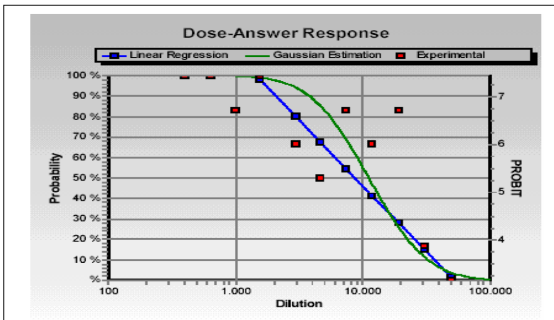
GRÁFICO 9 - Gráfico de dose-resposta para os Xilenos, segundo Modelo PROBIT , estabelecido por D. J. Finney .
