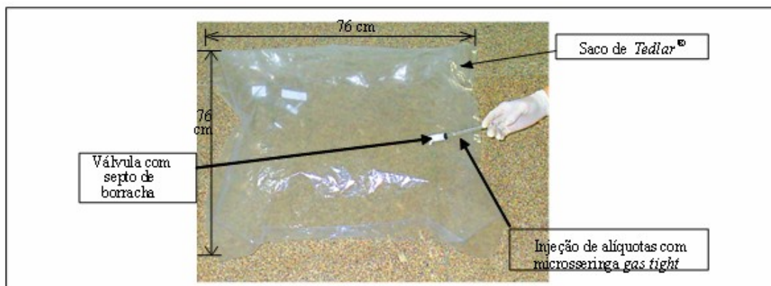
FIGURA 6 - Injeção dos compostos TEX nos sacos de Tedlar ® .
