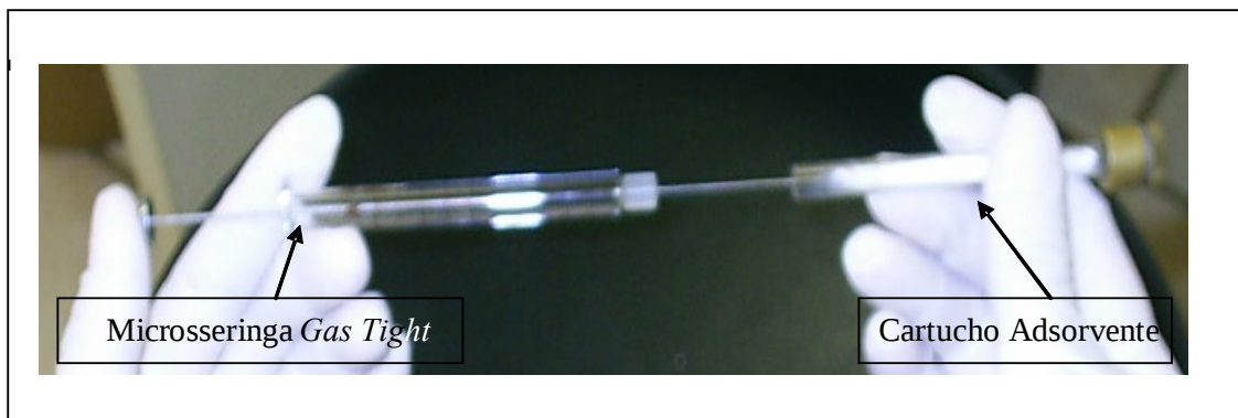
FIGURA 5 - Injeção de alíquota de solução-filha no cartucho adsorvente.
