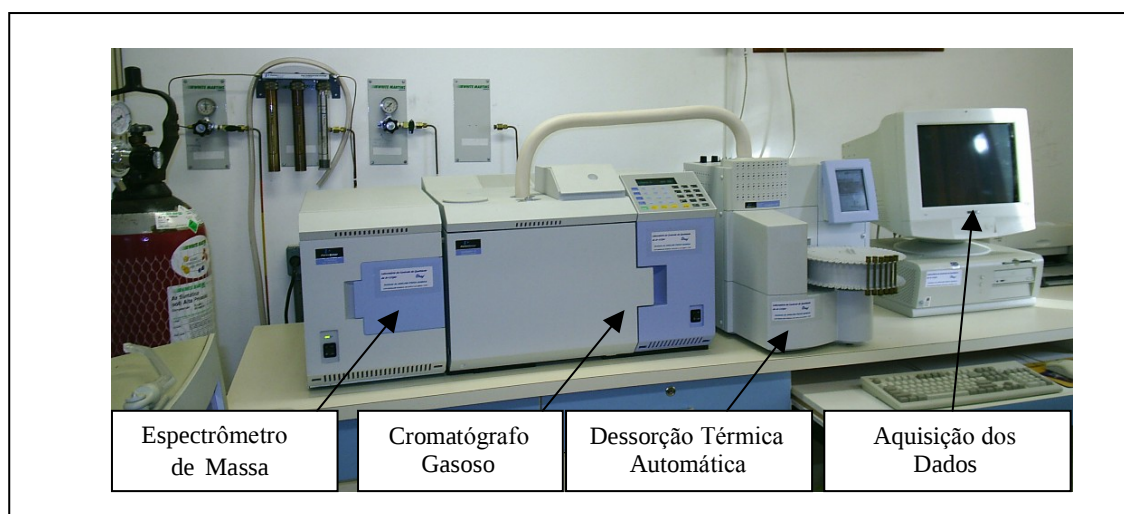
FIGURA 10 - Foto do sistema DTA-CG-EM do LCQAr.
