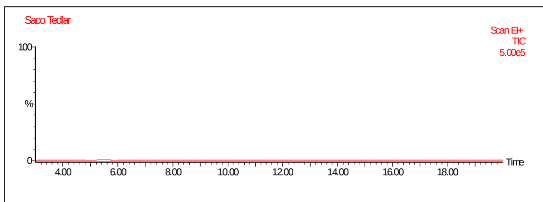
GRÁFICO 15 - Cromatograma de um saco de Tedlar ® após limpeza.
