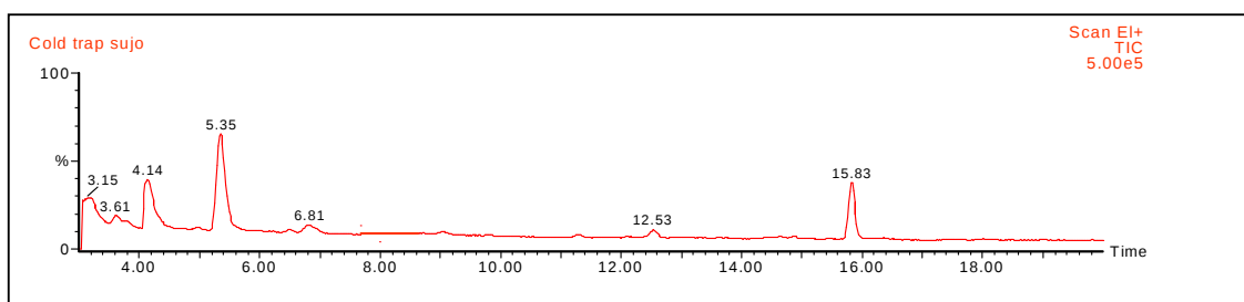
GRÁFICO 13 - Cromatograma do cold trap sujo, antes da limpeza.
