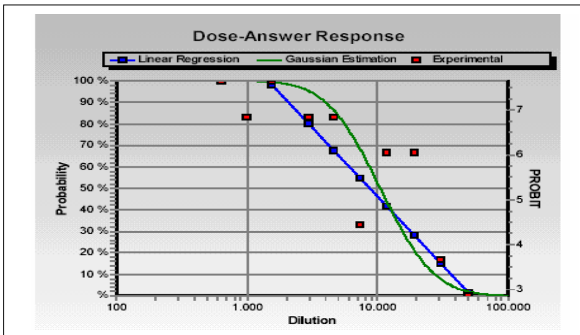
GRÁFICO 8 - Gráfico de dose-resposta para o Etilbenzeno, segundo Modelo PROBIT , estabelecido por D. J. Finney .
